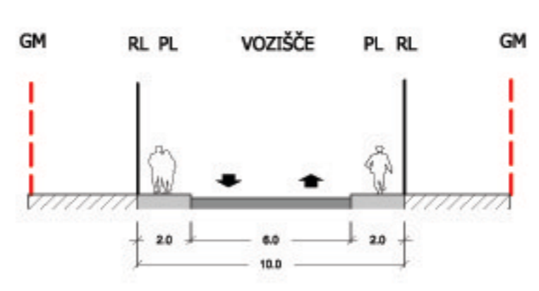
CESTNI PROFIL P3
