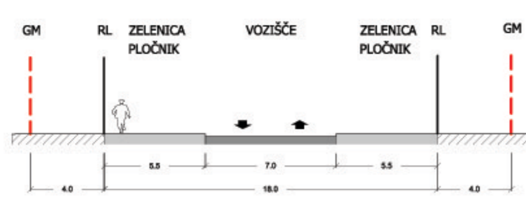
CESTNI PROFILI - merilo 1:200 CESTNI PROFIL P1
