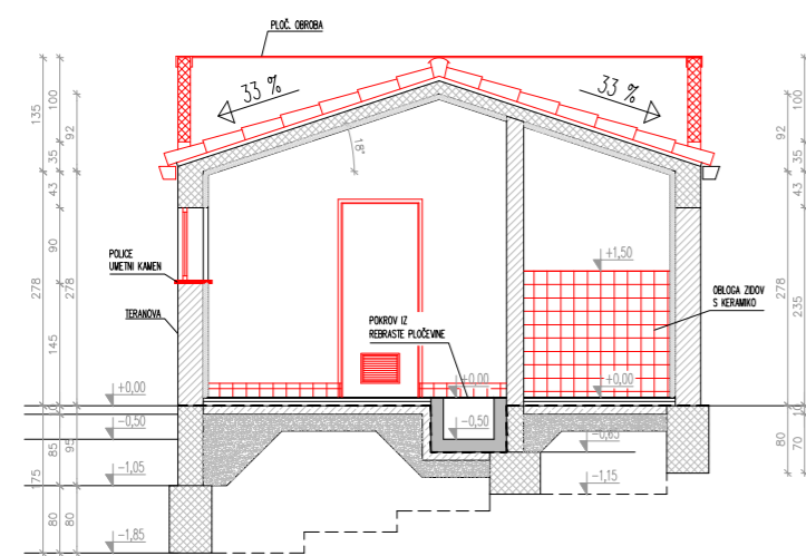
PREREZ A-A
