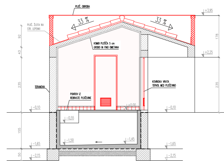
PREREZ C-C
