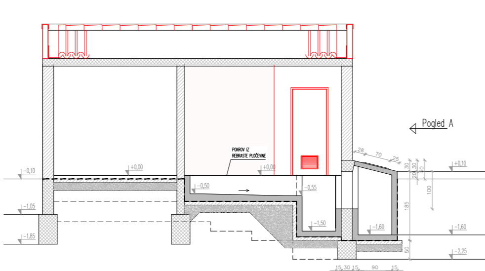
PREREZ D-D
