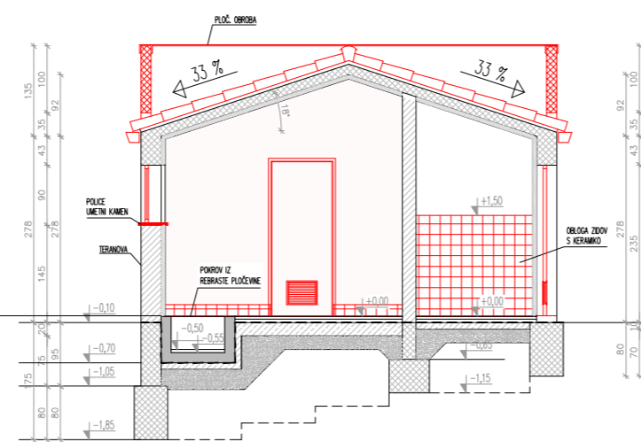
PREREZ B-B
